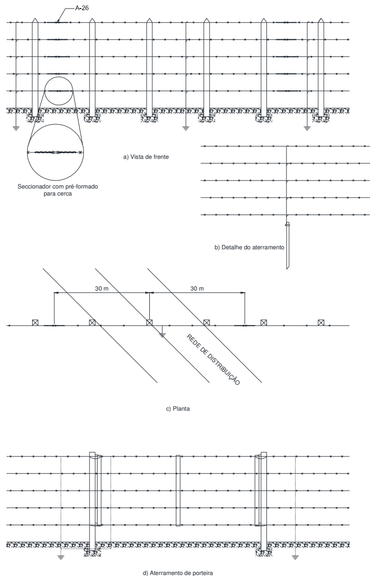
Figura 163 – Seccionamento de cerca – Cerca paralela
