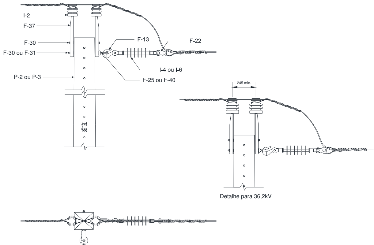
Figura 33 – Estrutura U3-2 – Poste de seção DT ou de madeira
