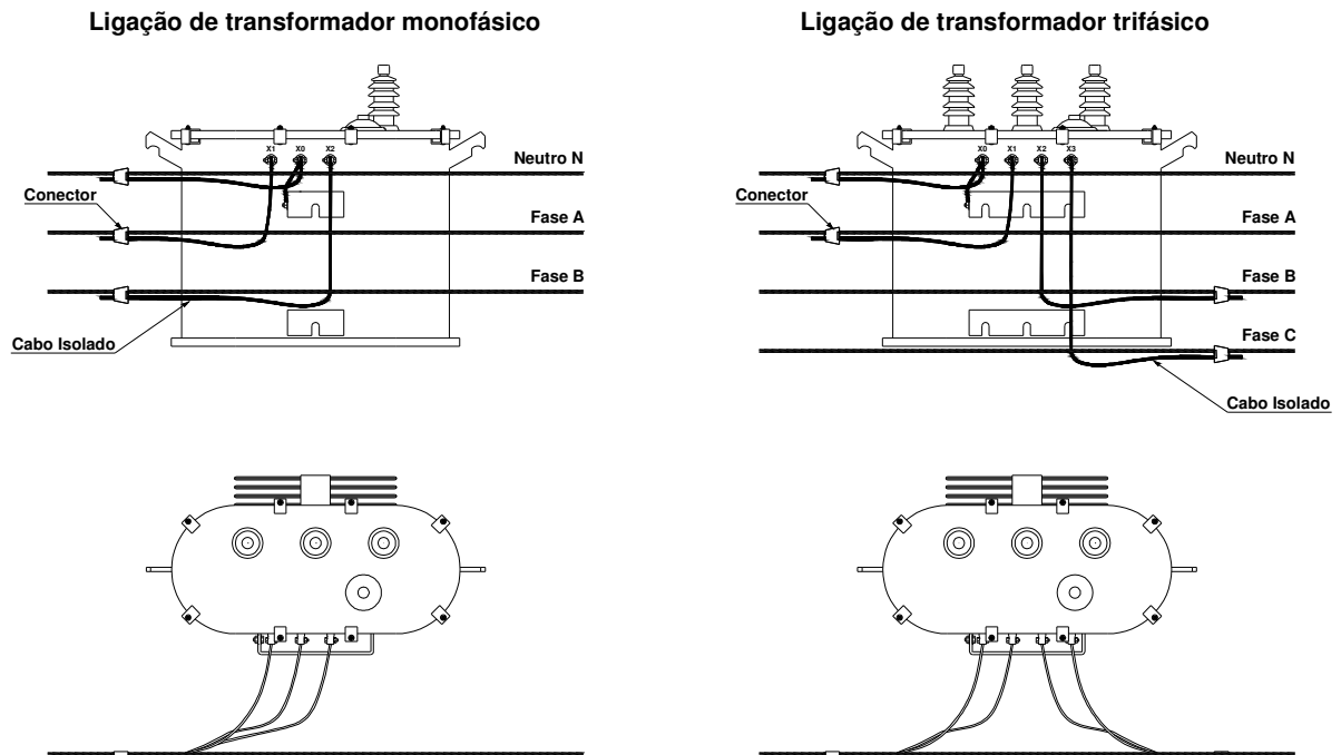
Figura 146 – Amarrações e ligações – Estrutura secundária – Ligação de baixa tensão do transformador
