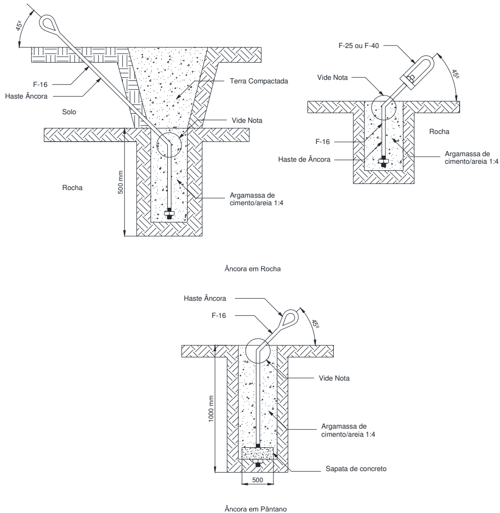
Figura 141 – Estai de âncora – Âncora em rocha e pântano
