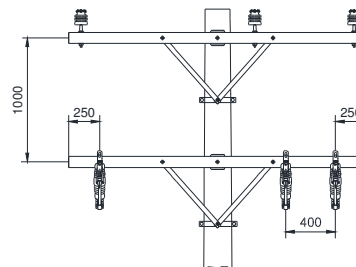
Normal - Cruzeta de 2400
