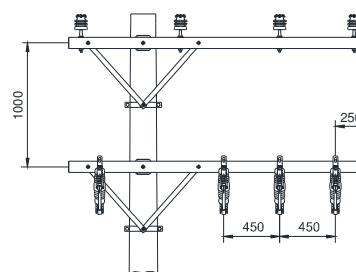
Meio beco - Cruzeta de 2400
