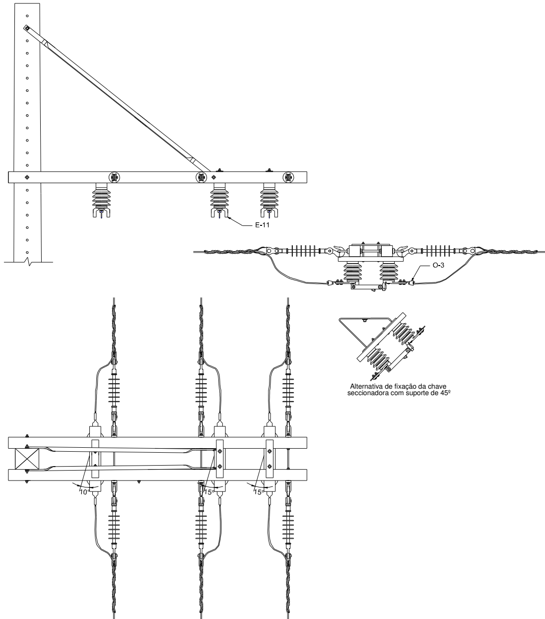
Figura 104 – Instalação de equipamento – Chave seccionadora – Estrutura trifásica B4
