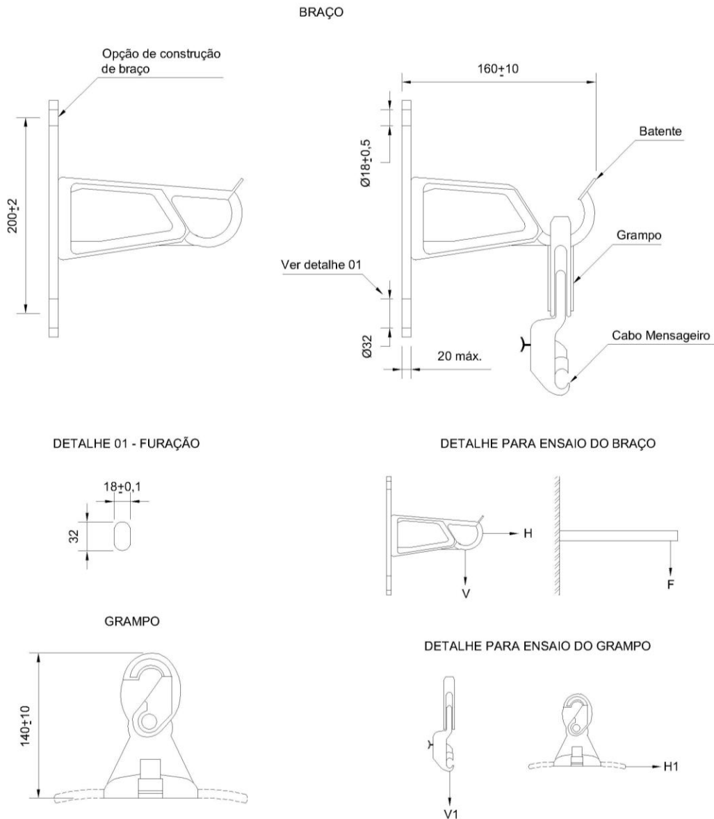
Figura 1 - Desenho dimensional conjunto grampo de suspensão
