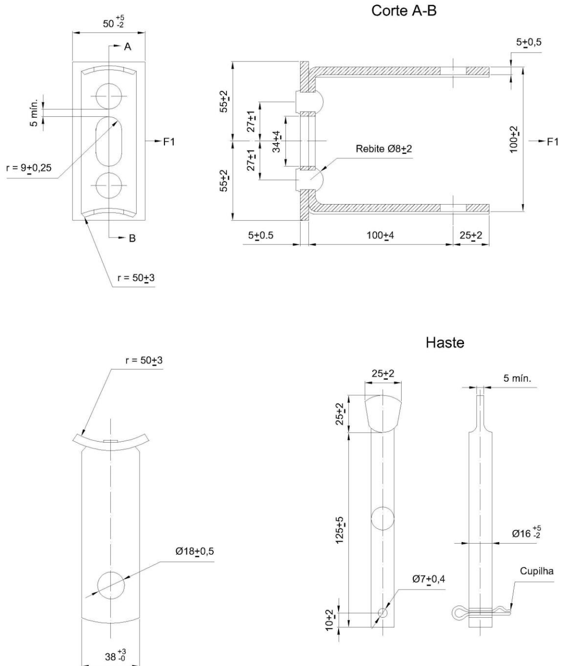
Figura 6 - Desenho dimensional armação secundária de 1 estribo
