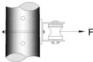
Figura 7 - Desenho dimensional isolador roldana
