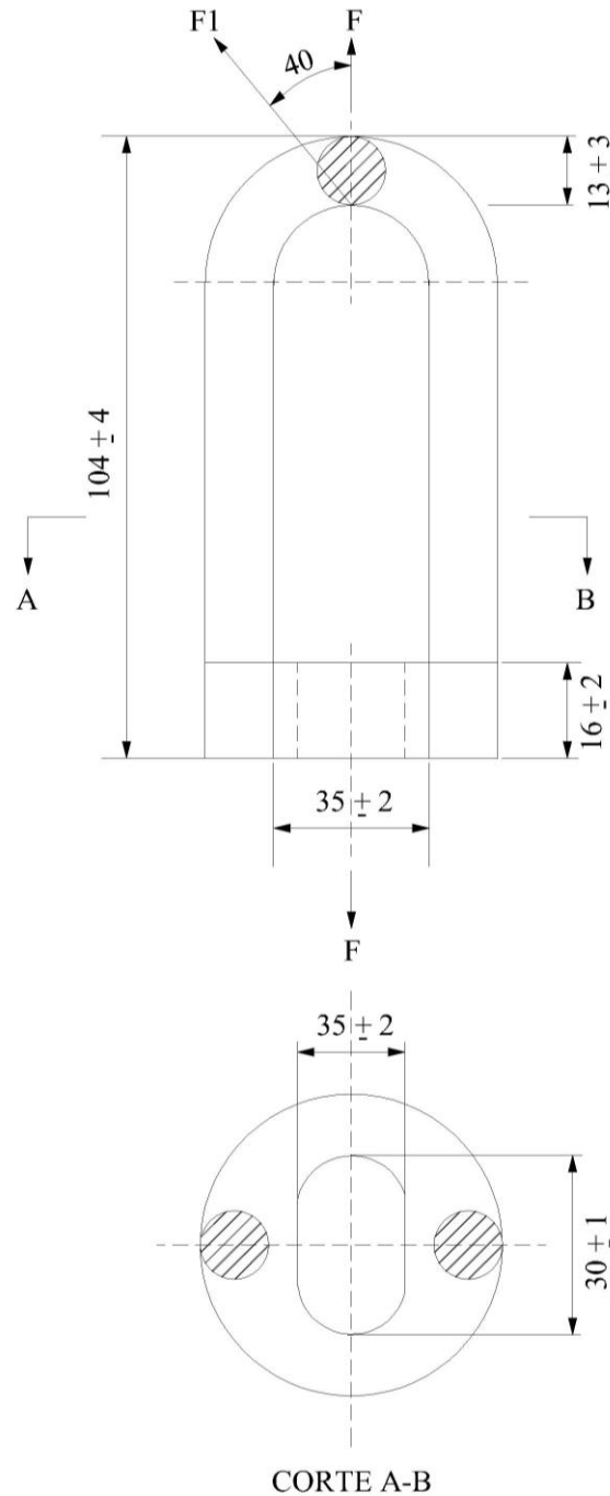
Figura 2 - Desenho dimensional olhal para parafuso
