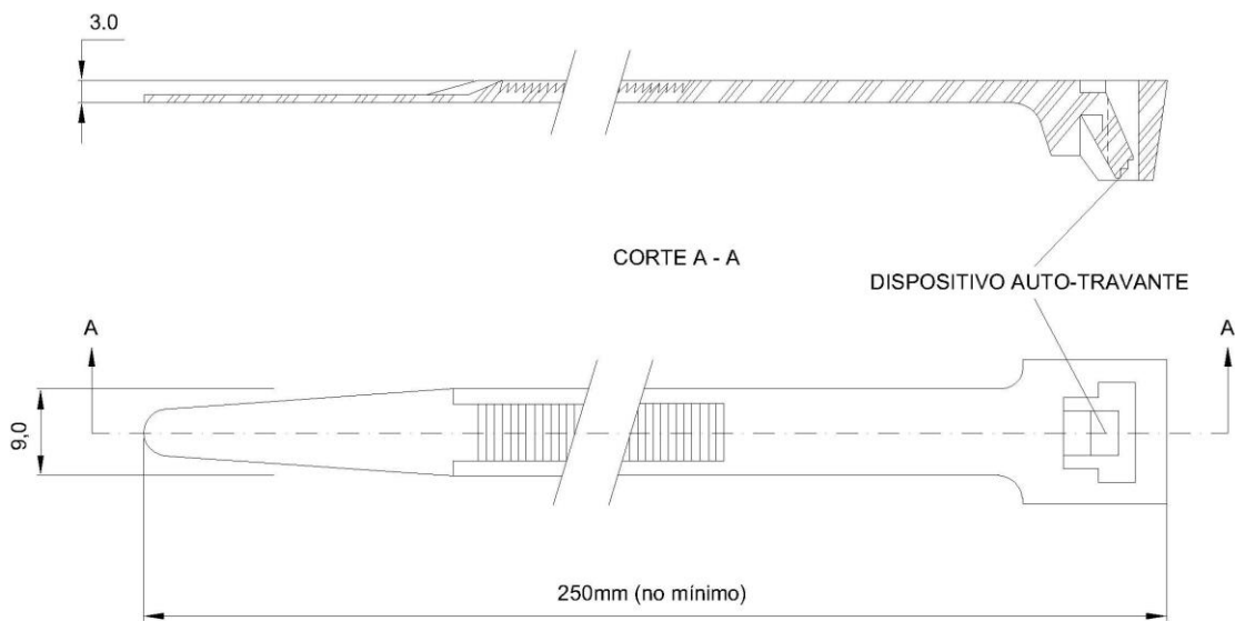
Figura 4 - Desenho dimensional braçadeira plástica
