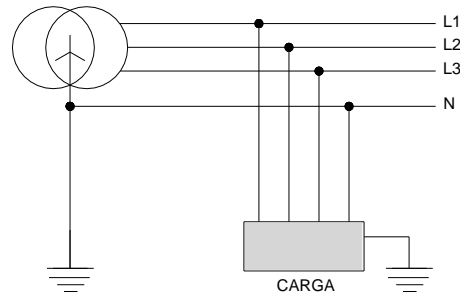
Figura 4 - Esquema TT
